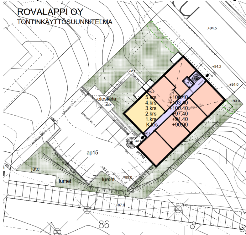
Kuva 8. Asemapiirustus arkkitehtisuunnittelu Hiilivirta Oy vaihtoehto 1
